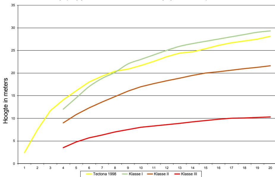
Vergelijking groei Tectona - Site klassen Keogh gedurende 20 jaar
